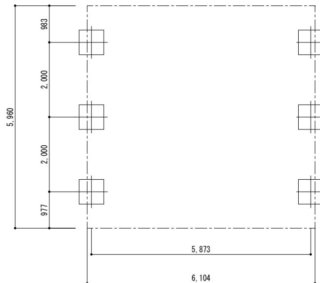
■ 基礎配置図
